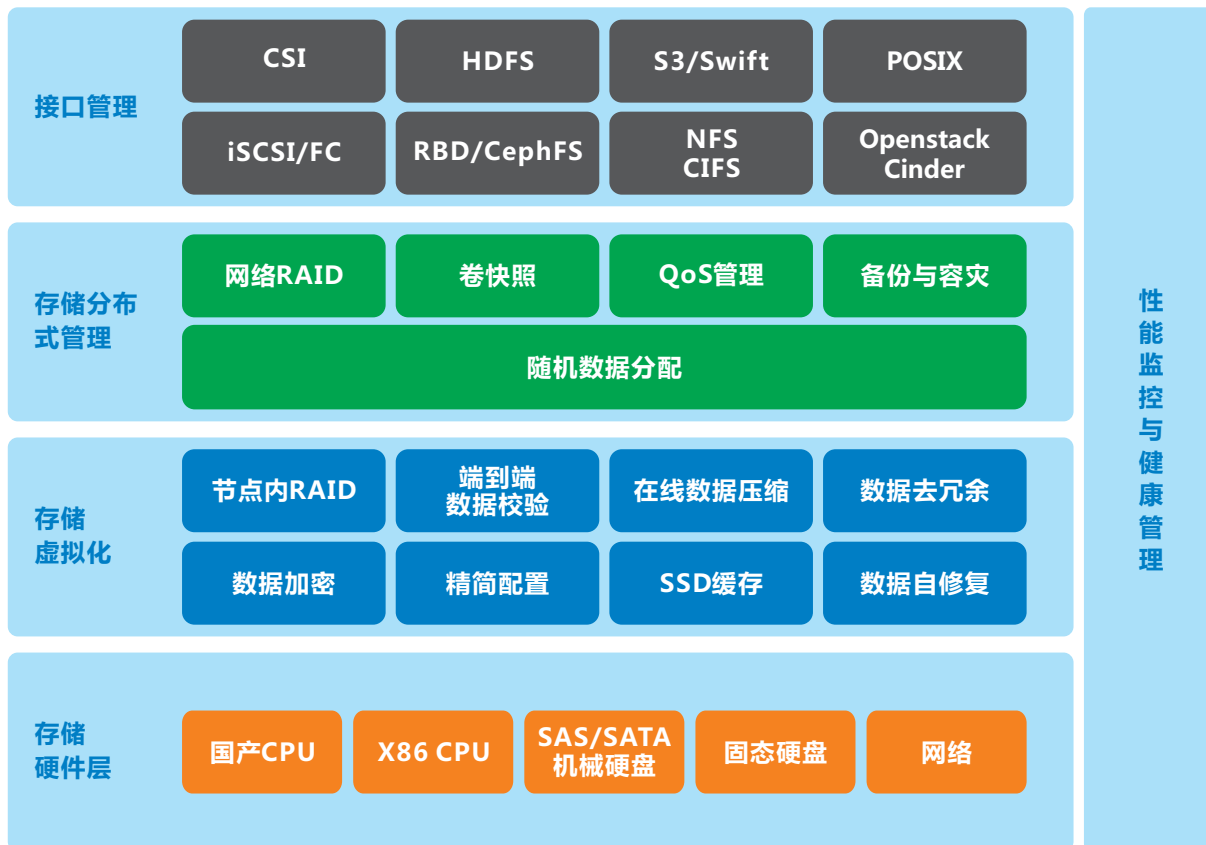
Titlis分布式存储架构图
